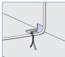
3 バインド線等でケーブルを支持します。
