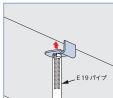
2 梁部に貼付けます。パイプを使えば脚立なしで施工可能です。
