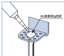
1 当社接着剤 (MJ 接着剤) を塗布します。
