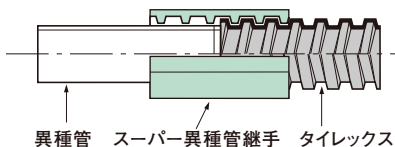
異種管 スーパー異種管継手 タイレックス
