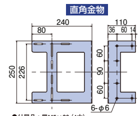
直角金物
