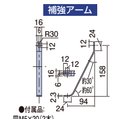
補強アーム
