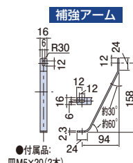
補強アーム
