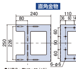
直角金物
