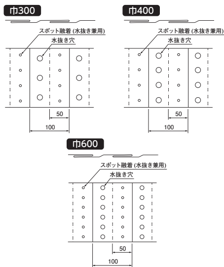
折込み構造図
