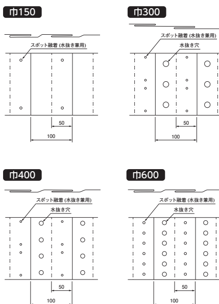
折込み構造図
