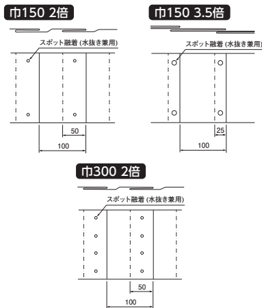
折込み構造図
