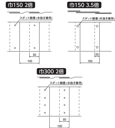
折込み構造図
