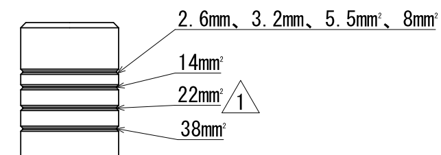
打込み確認線 適用電線サイズ
