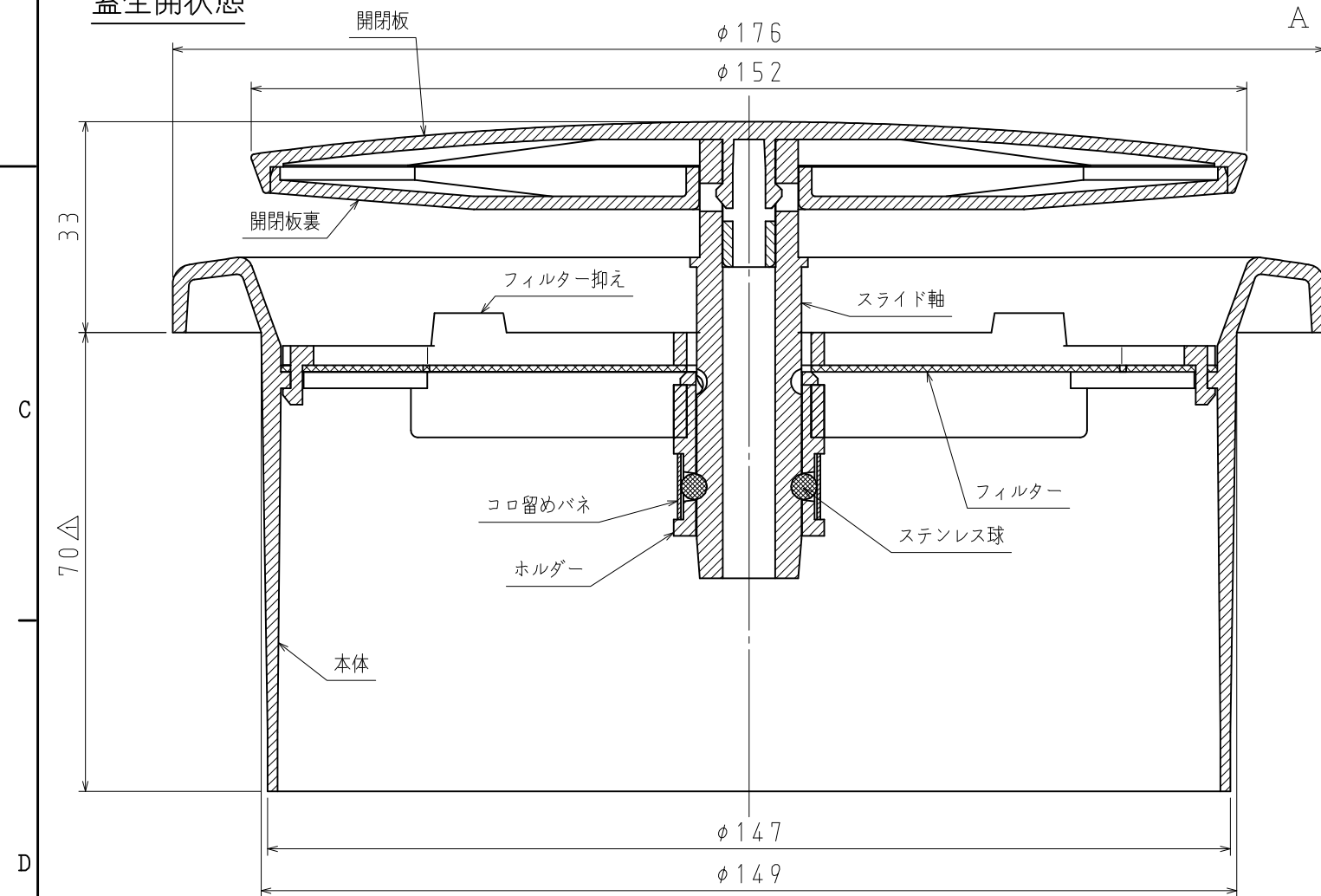
蓋全開状態
