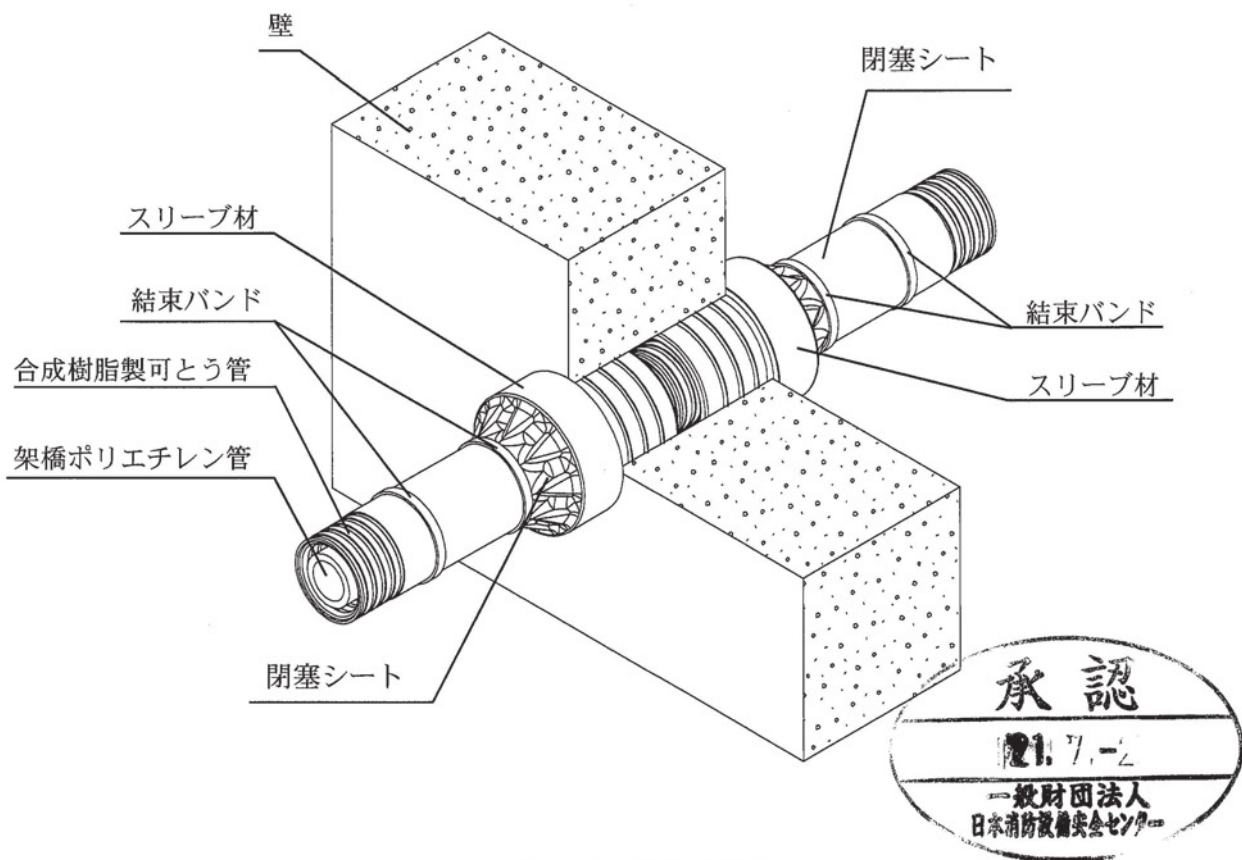
図-2 構造斜視図
