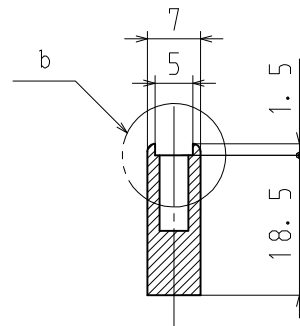
A-A断面図
