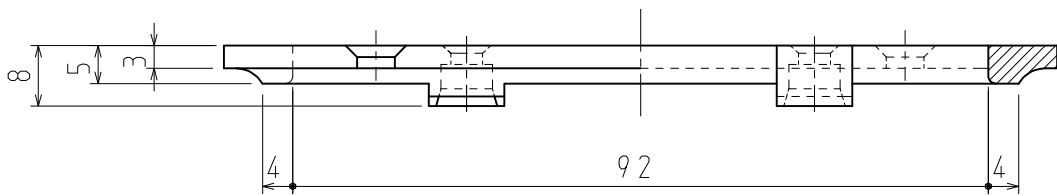
A-A断面図
